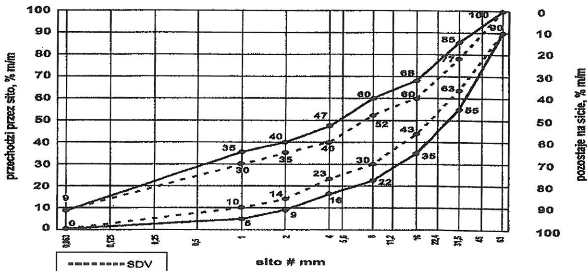
Rys. 1. Krzywe graniczne uziarnienia mieszanki kruszywa niezwiązanej 0/63 mm
