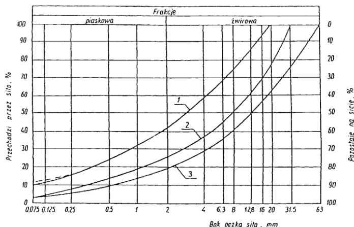
Rysunek 1. Pole dobrego uziarnienia kruszyw przeznaczonych na podbudowy wykonywane metodą stab. mechanicznej
