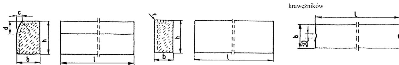
Rys. 1. Wymiarowanie krawężników
