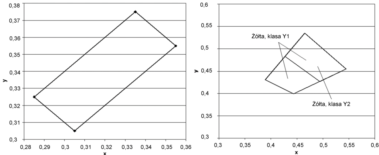
Rys. 3. Granice barw białej, żółtej, czerwonej, niebieskiej i zielonej oznakowania
